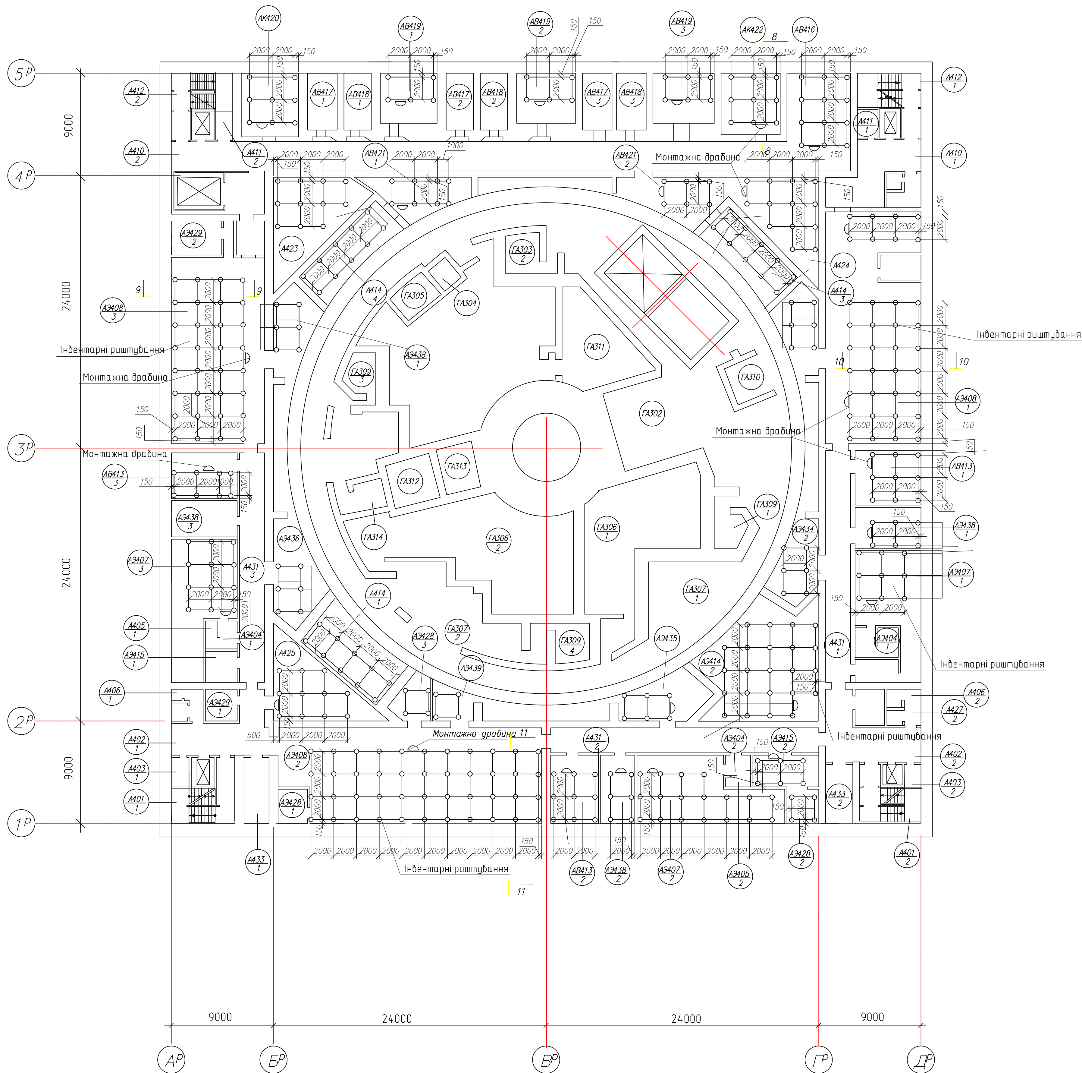
Схема влаштування інвентарних трубчатих риштувань на відмітці 13,200
